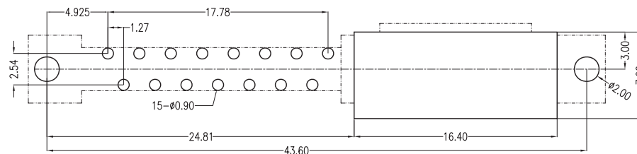
P.C.B. Layout(T=3.0)
