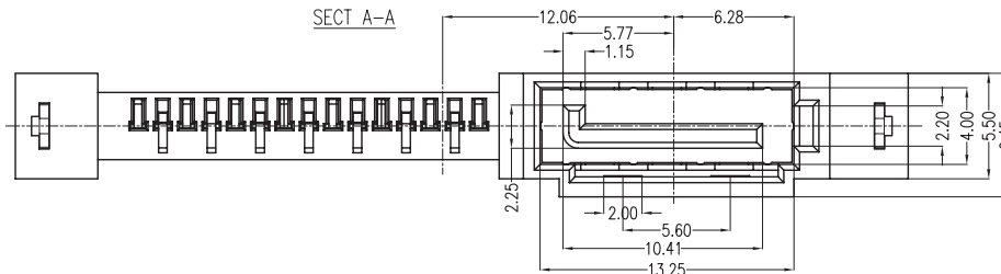
SECT A-A
