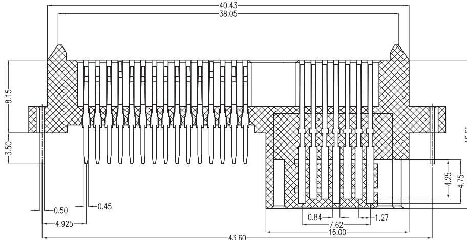
SECT A-A
